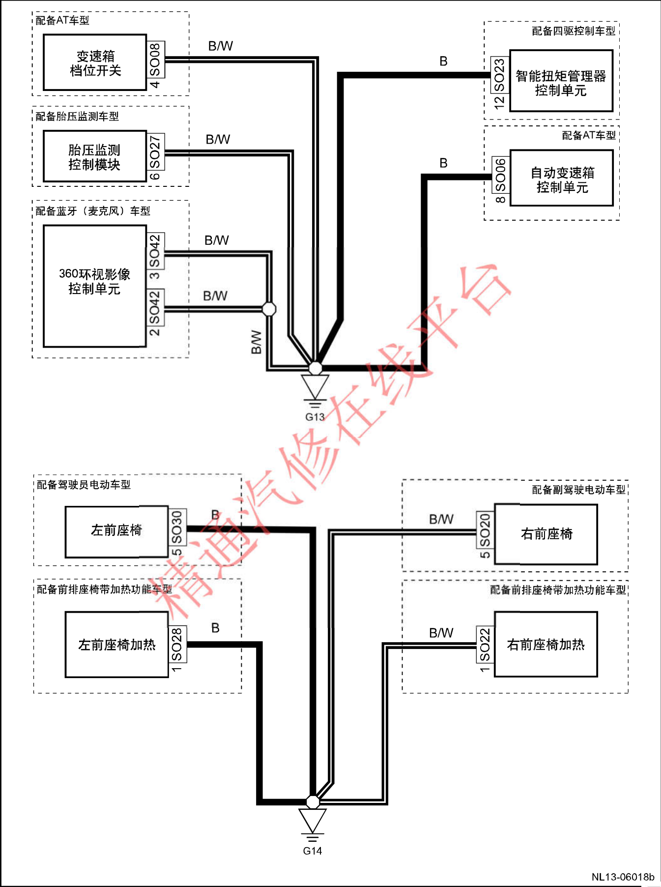
接地线路图8 ( G13,G14 )
