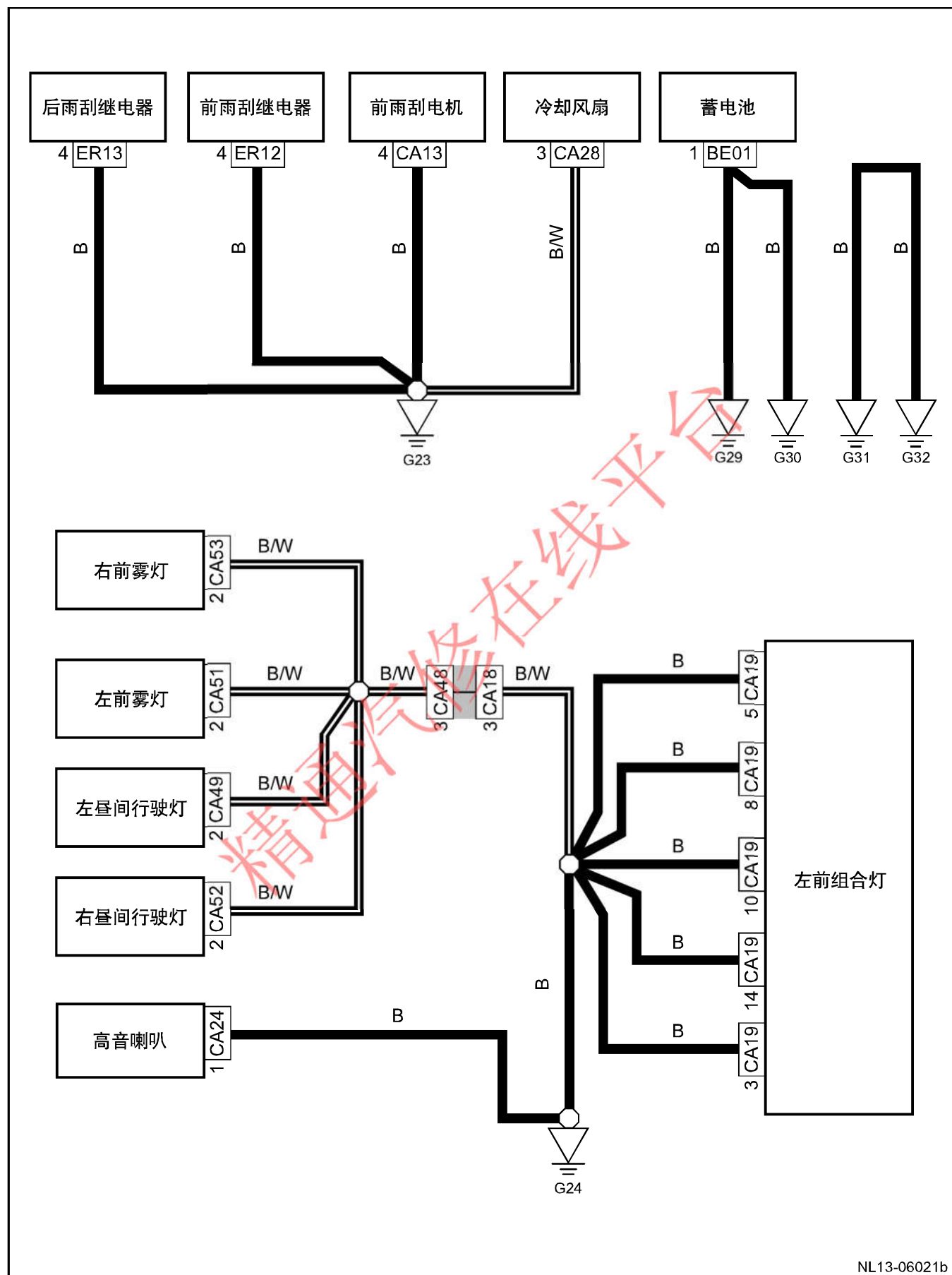
接地线路图11 ( G23,G24,G29,G30,G31,G32 )
