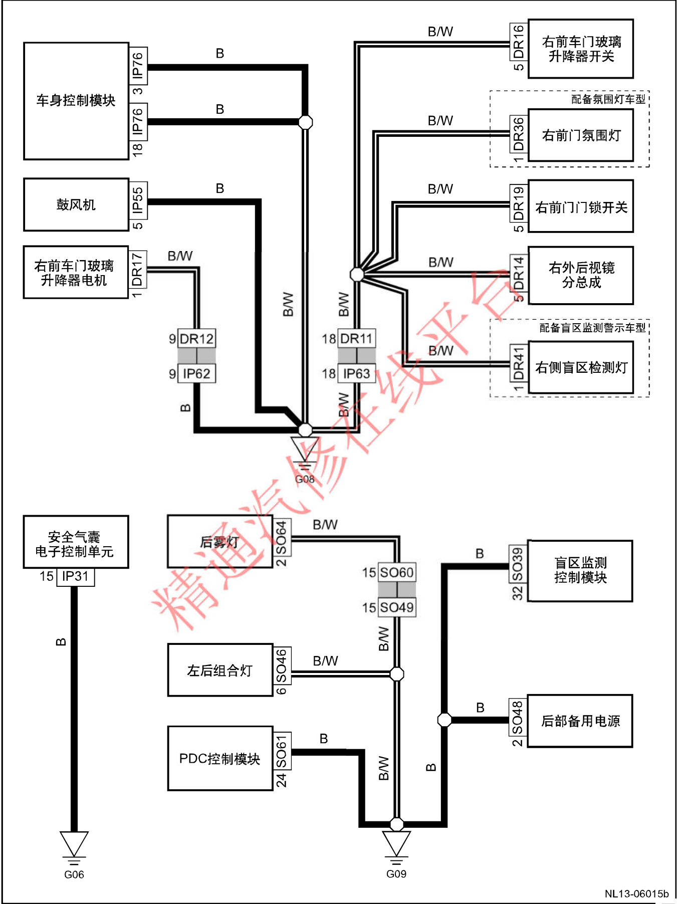
接地线路图5 ( G06,G08,G09 )
