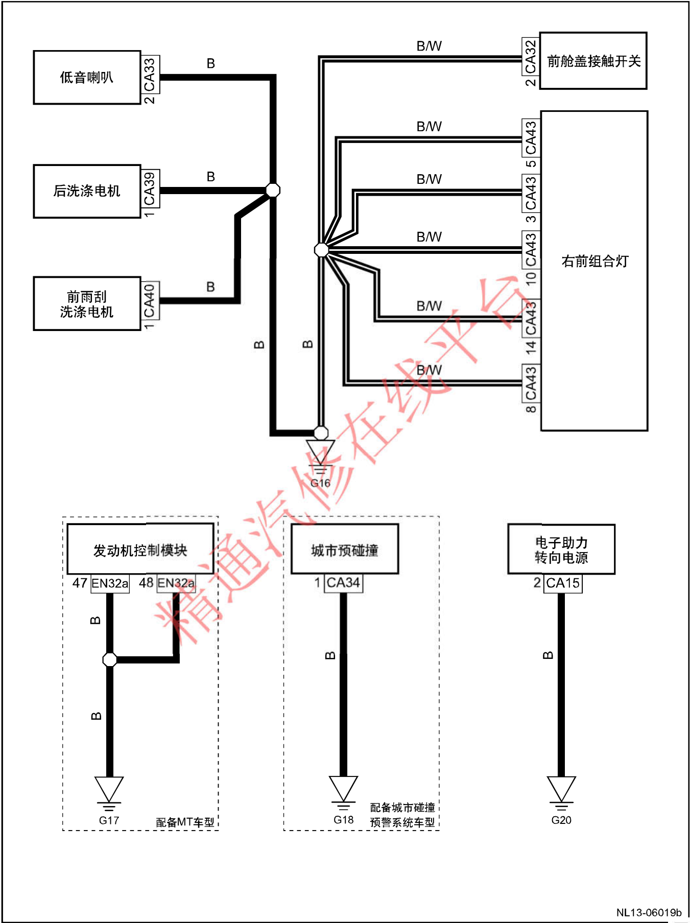
接地线路图9 ( G16,G17,G18,G20 )
