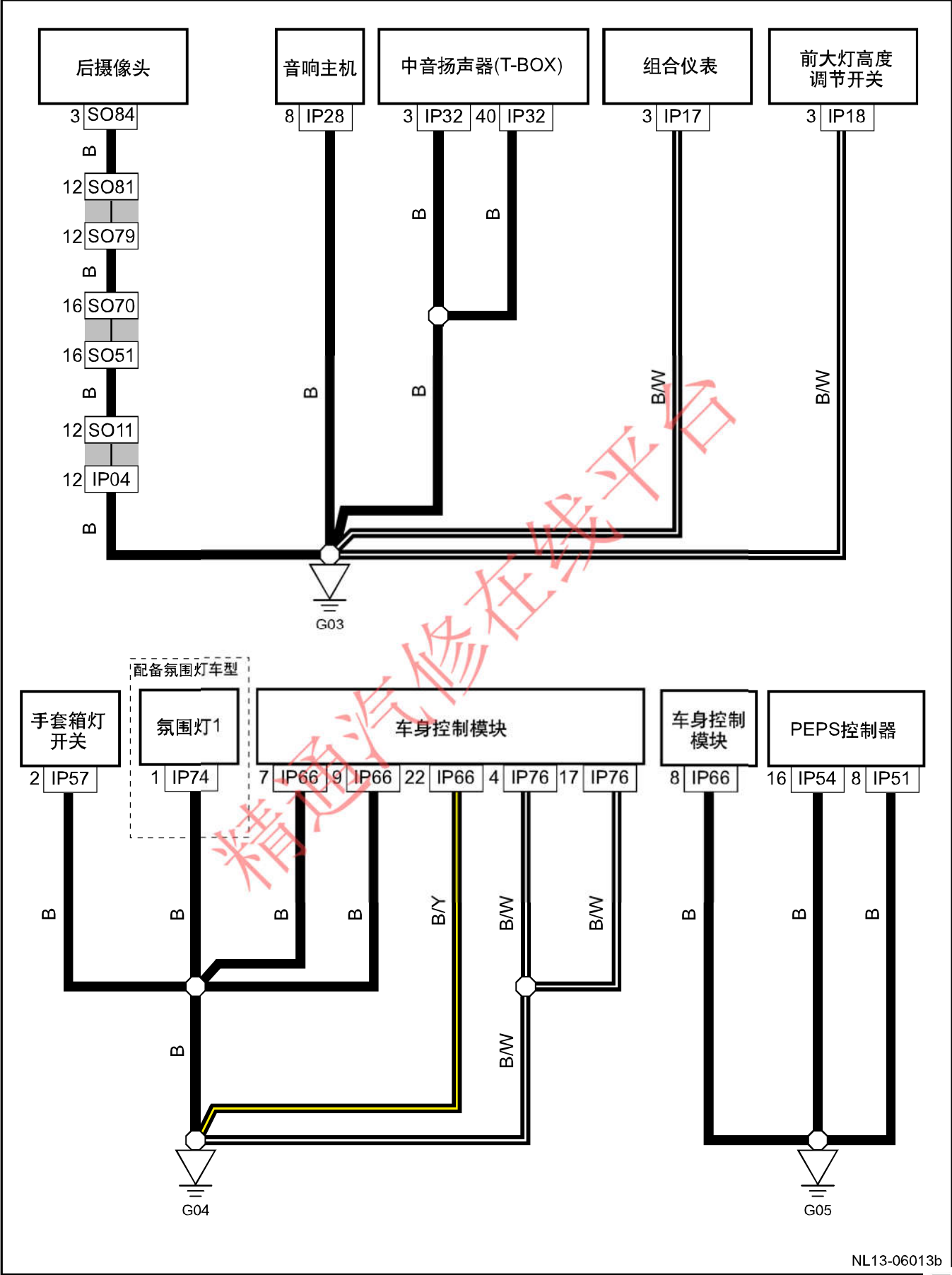
接地线路图3 ( G03,G04,G05 )
