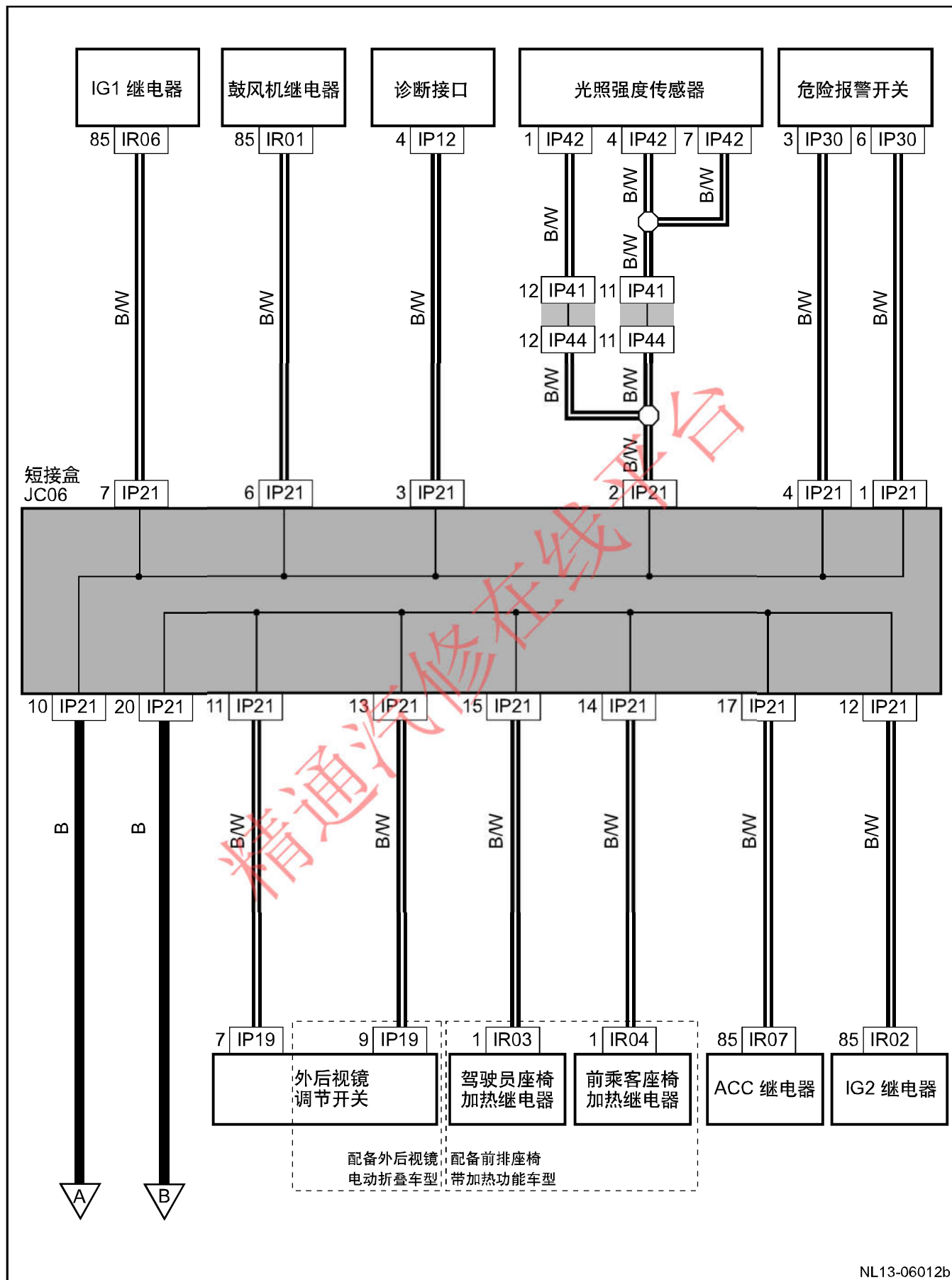
接地线路图2 ( G01续 )
