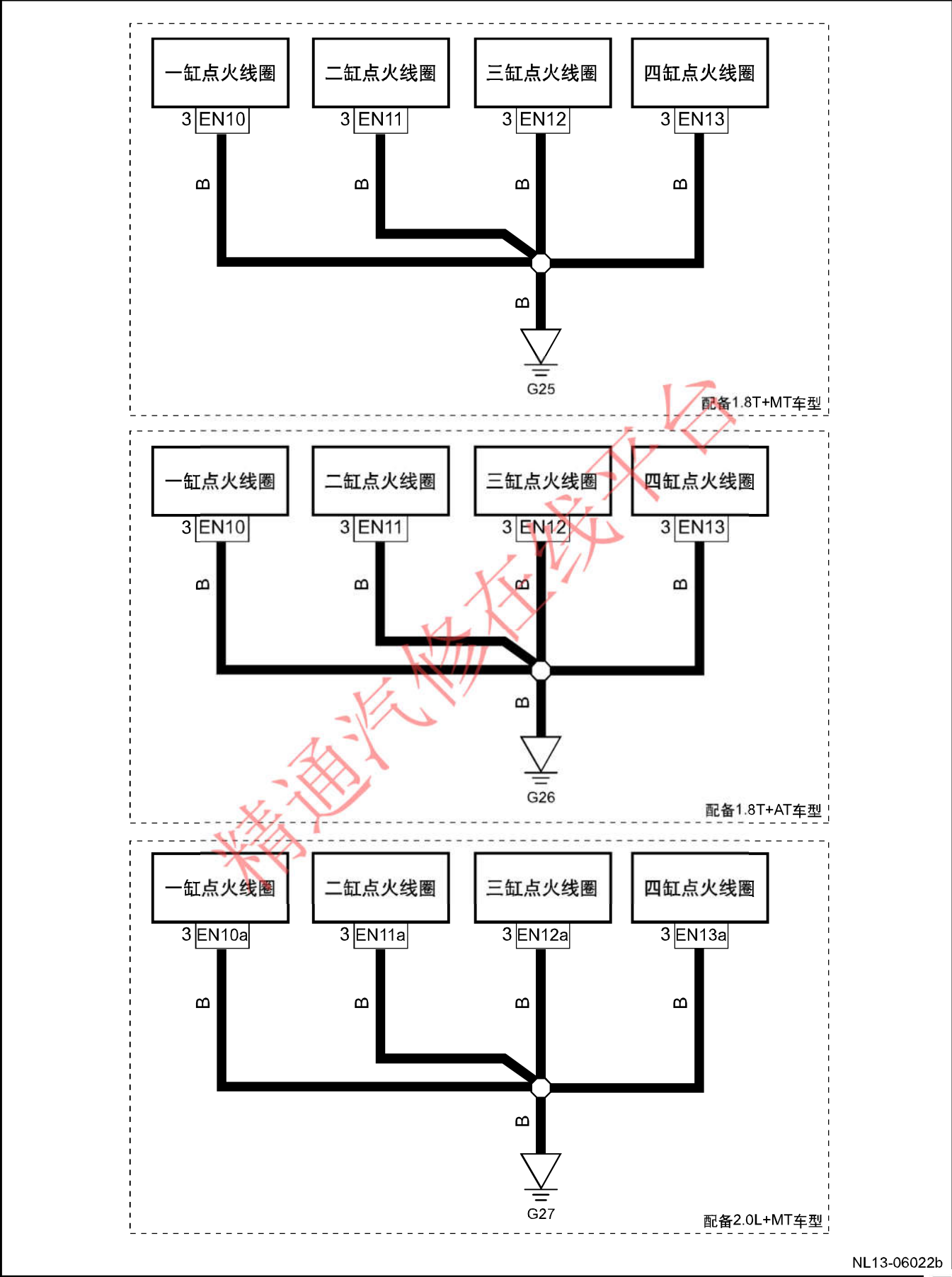
接地线路图12 ( G25,G26,G27 )
