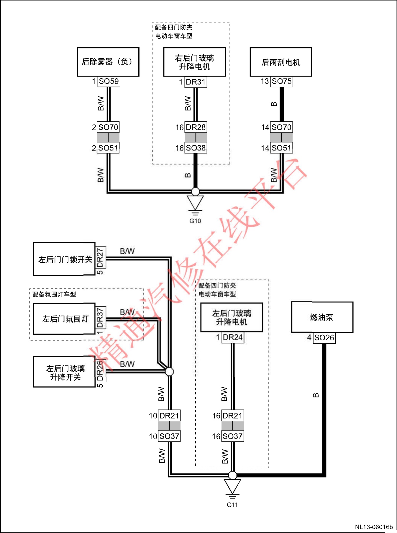
接地线路图6 ( G10,G11 )
