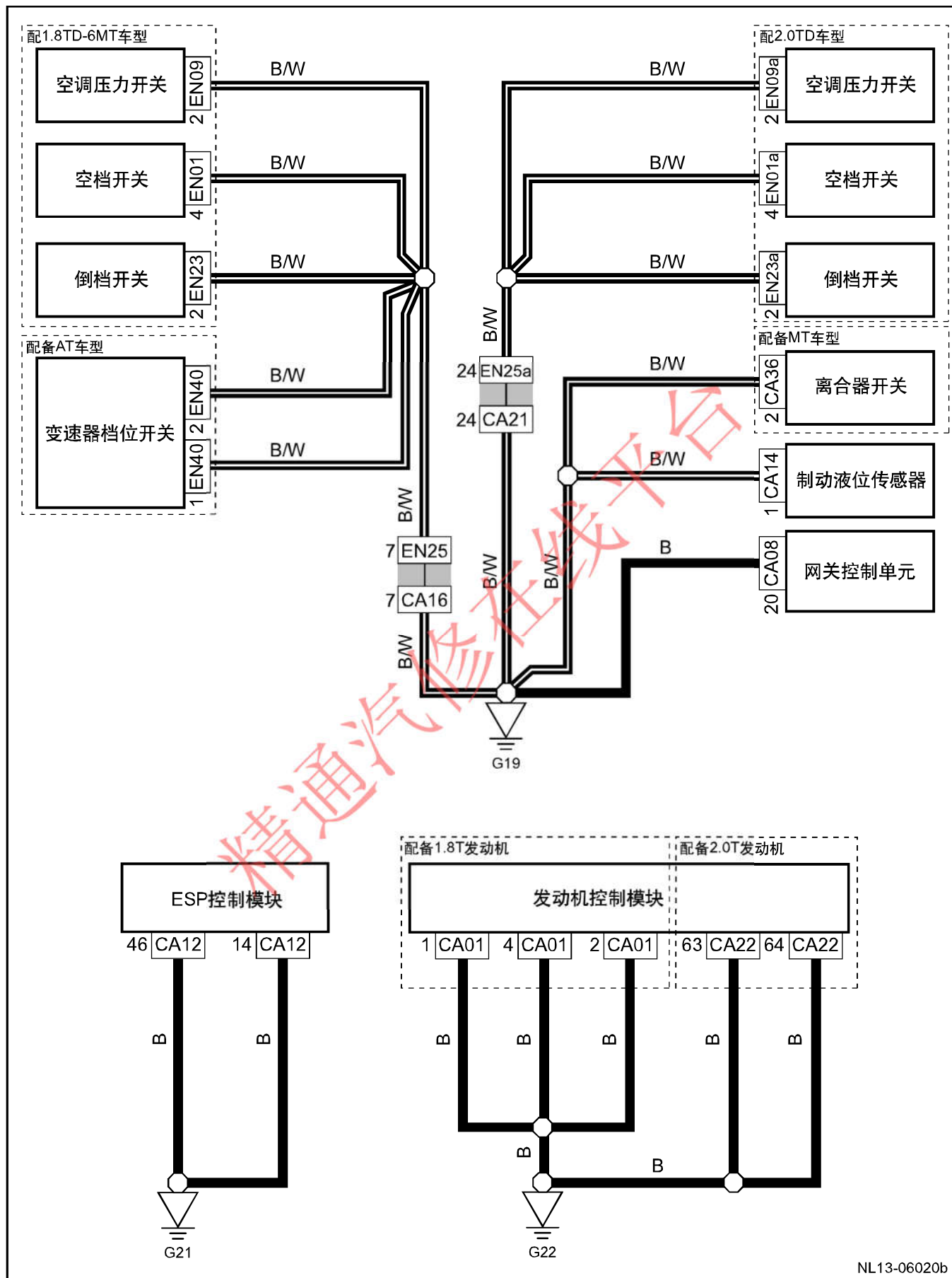
接地线路图10 ( G19,G21,G22 )
