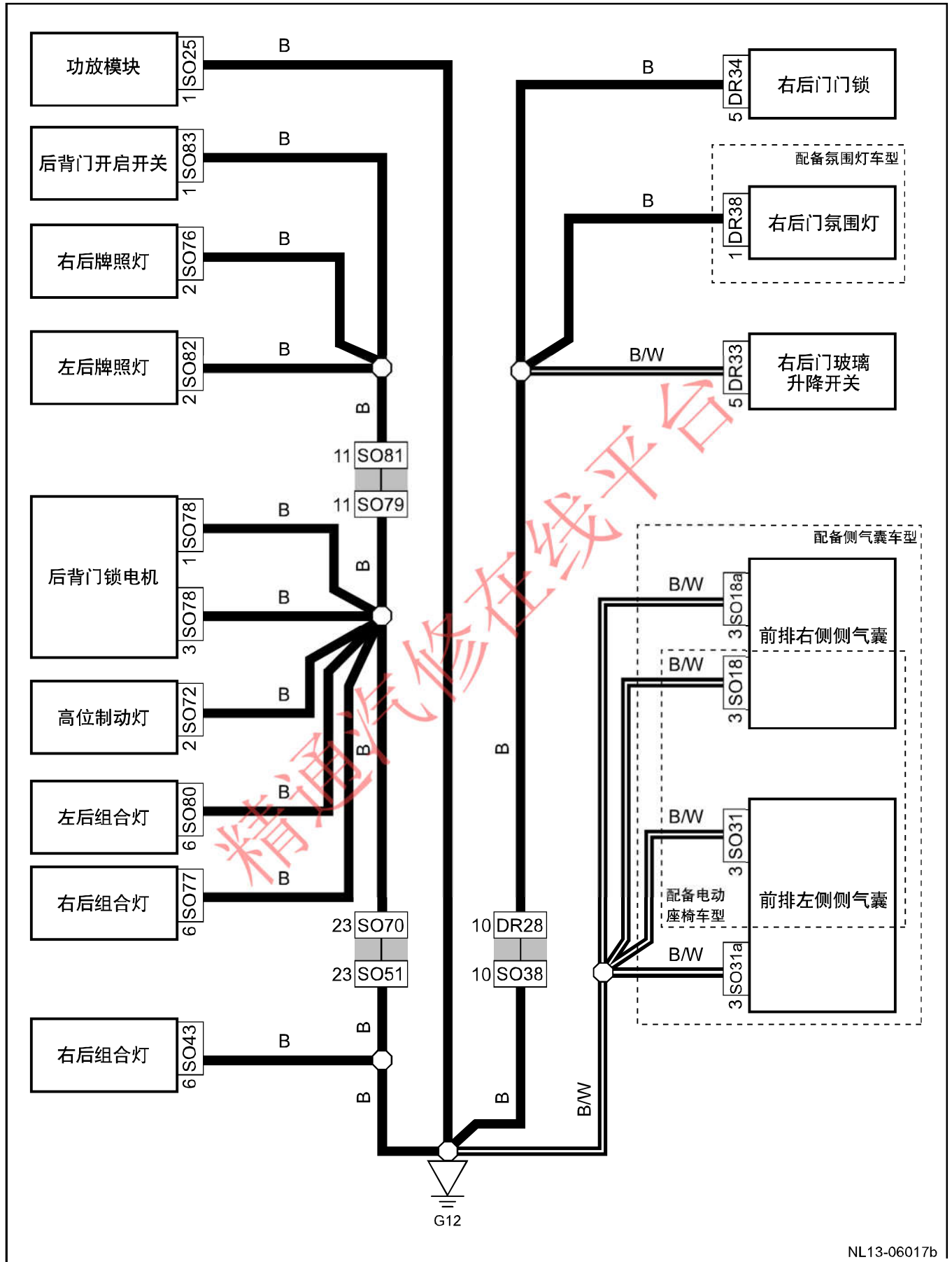
接地线路图7 ( G12 )
